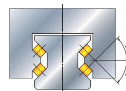
剖面图
